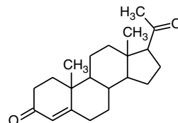
Progesterone
