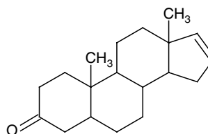
Androstene
