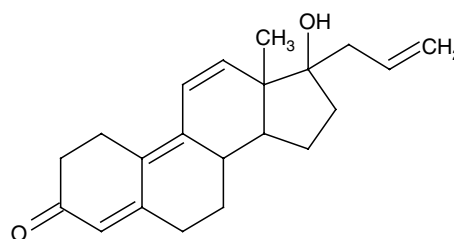
Altrenogest
