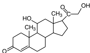
Corticosterone
