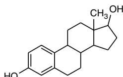
Oestradiol
