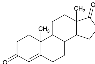
4-Androsten-3,17-dione
