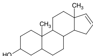
Androstene
