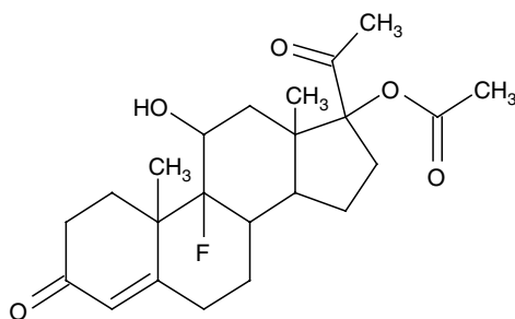
Fluogestone acetate
