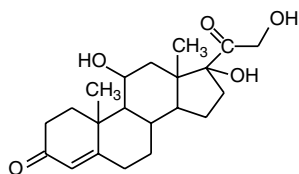
Cortisol
