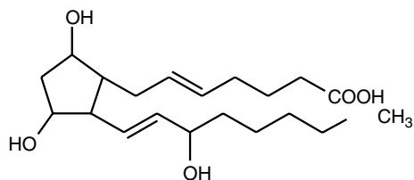
PGF 2α
