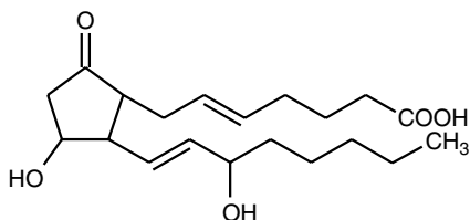
PGE 2
