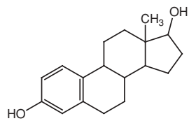
17-β-estradiol
