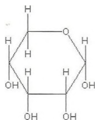
ribose
