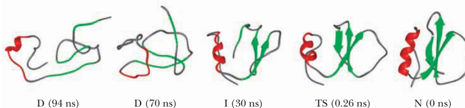
Cl2
