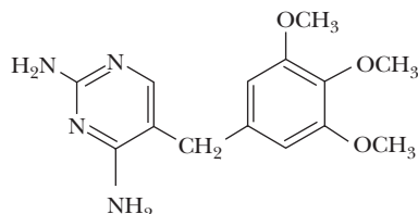
Trimethoprim
