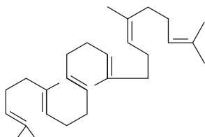
Squalene
