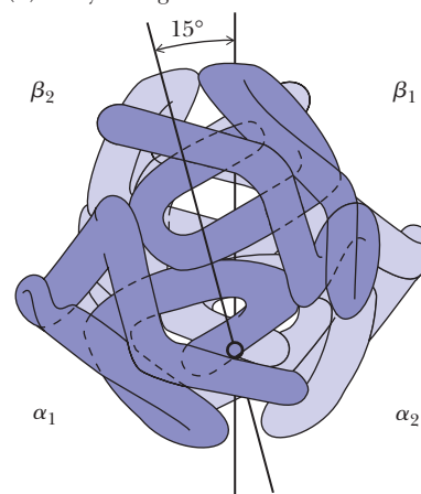
(b) Oxyhemoglobin
