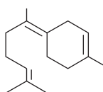
Bisabolene
