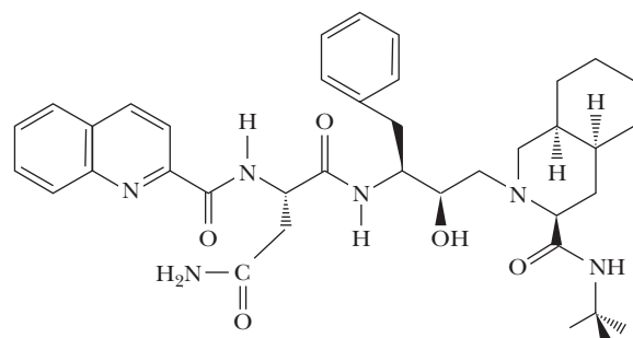
Invirase (saquinavir)
