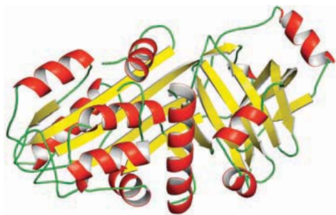
Ovalbumin monomer
